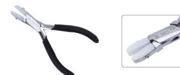
型号 Model: T.SPS380FF 总长度 Total length: 125mm 重量 Weight: 75g/Pcs
