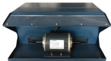
双头吸尘打磨机 Double heads dust collection grinding machine
