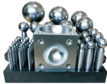
特大窝珠作套装 Dapping bead
